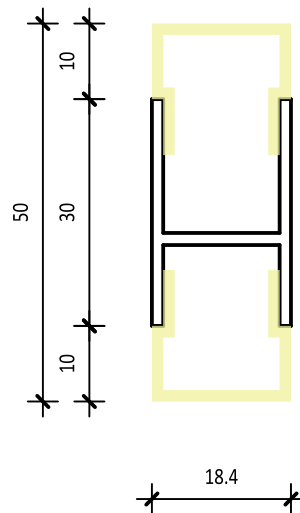
Diffusor HOCH/HOCH
