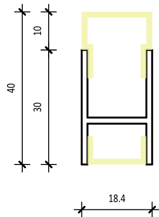
Diffusor HOCH/FLACH
